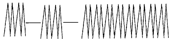
c) Missing Cycle MCY 1:8
